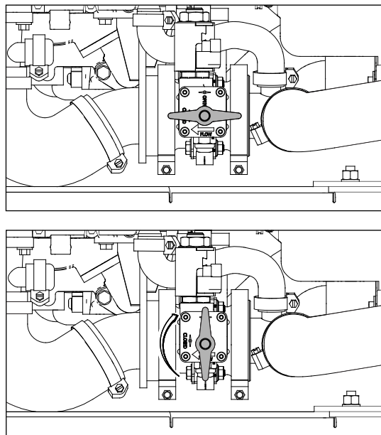
Figure 4-3. Réinitialisation du robinet ASOV (de la position ouverte à fermée)
