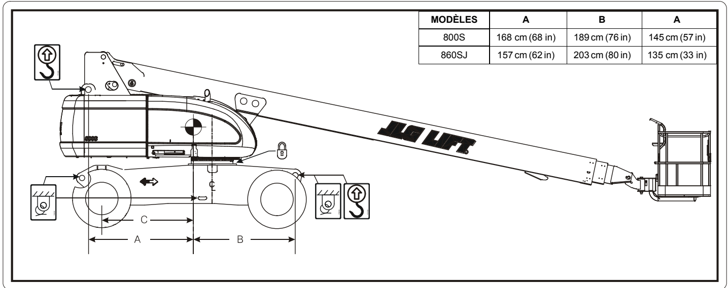
Figure 4-8. Tableau de levage et d'arrimage
