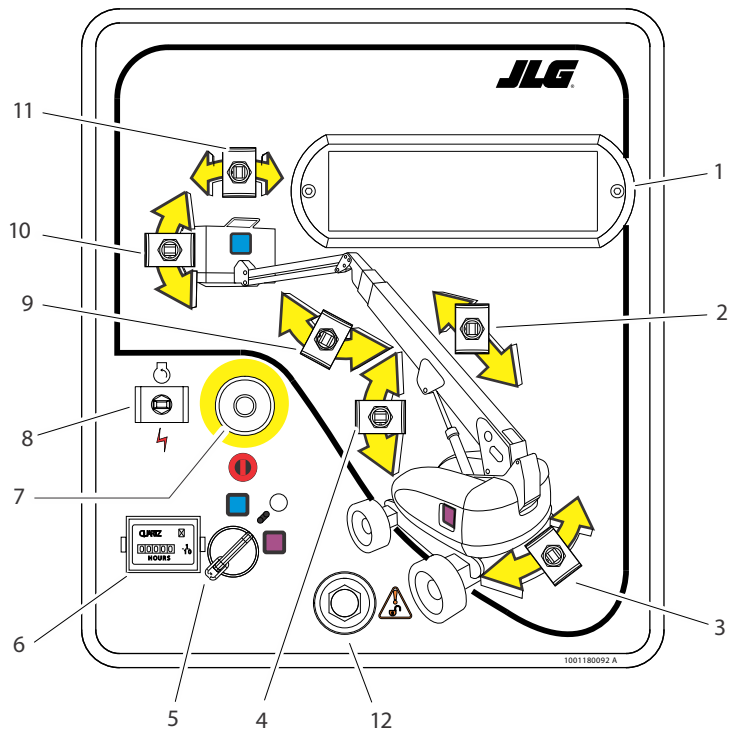
Figure 3-5. Console de commande au sol – 860SJ avec MSSO
