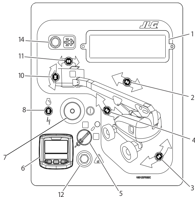
Figure 3-3. Console de commande au sol – 800S avec MSSO et FAP
