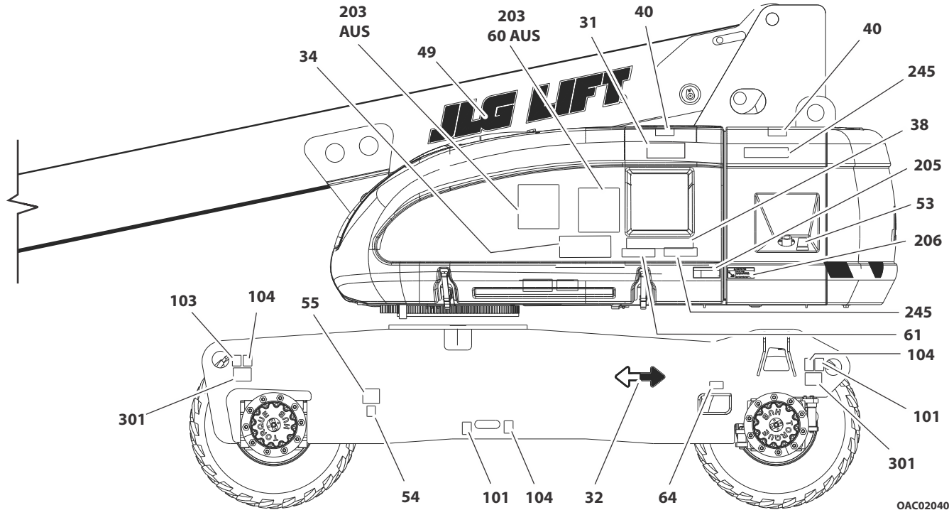
Figure 4-10. Emplacement des autocollants – Emplacement des autocollants, 800S, Fiche 2 de 5
