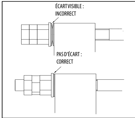
Figure 6-2. Tension du câble antichute externe boulonné
