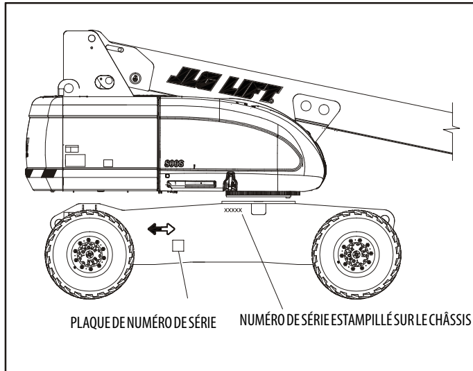
Figure 7-1. Emplacements du numéro de série
