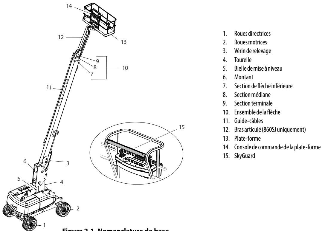
Figure 2-1. Nomenclature de base
