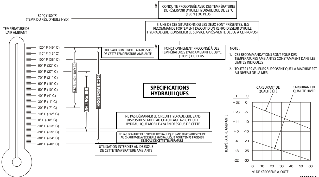
Figure 7-3. Caractéristiques de température de fonctionnement du circuit hydraulique – Deutz – Fiche 2 de 2
