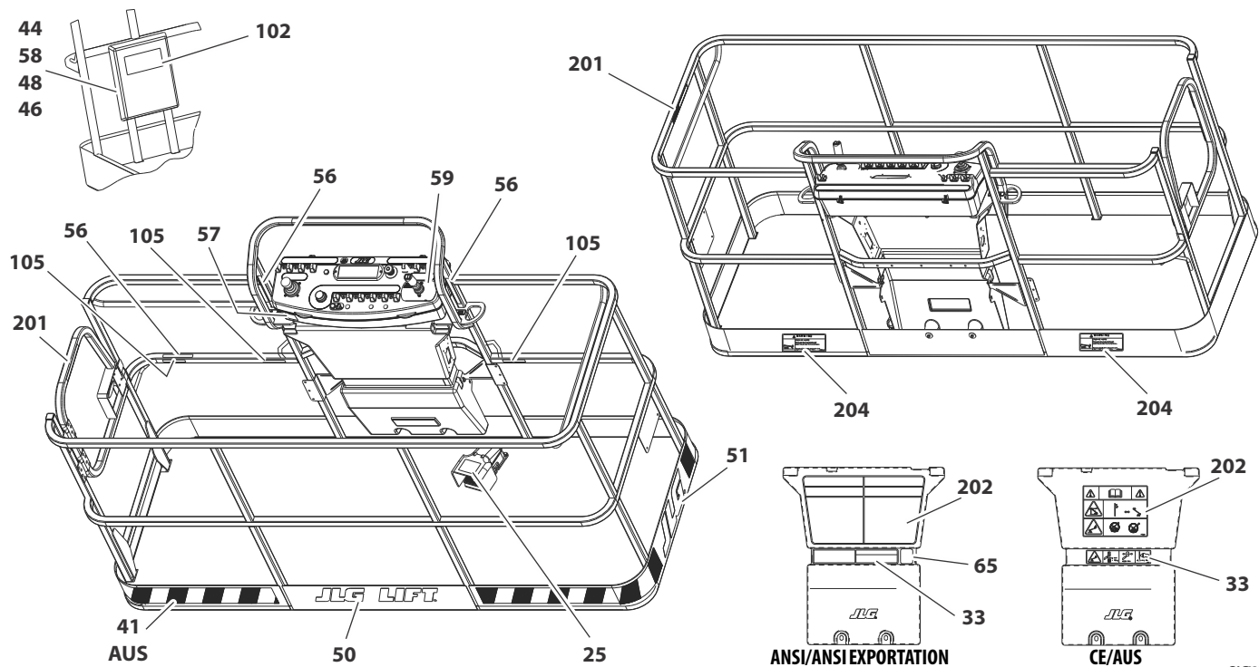
Figure 4-13. Emplacement des autocollants – Emplacement des autocollants, 800S, Fiche 5 de 5
