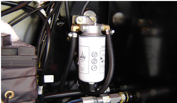
B. Filtre à carburant – Deutz TD 2,9 I (sur le réservoir hydraulique)
