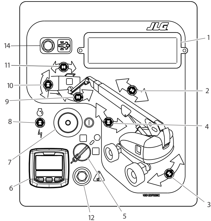
Figure 3-6. Console de commande au sol – 860SJ avec MSSO et FAP
