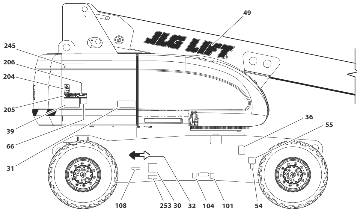
Figure 4-9. Emplacement des autocollants – Emplacement des autocollants, 800S, Fiche 1 de 5
