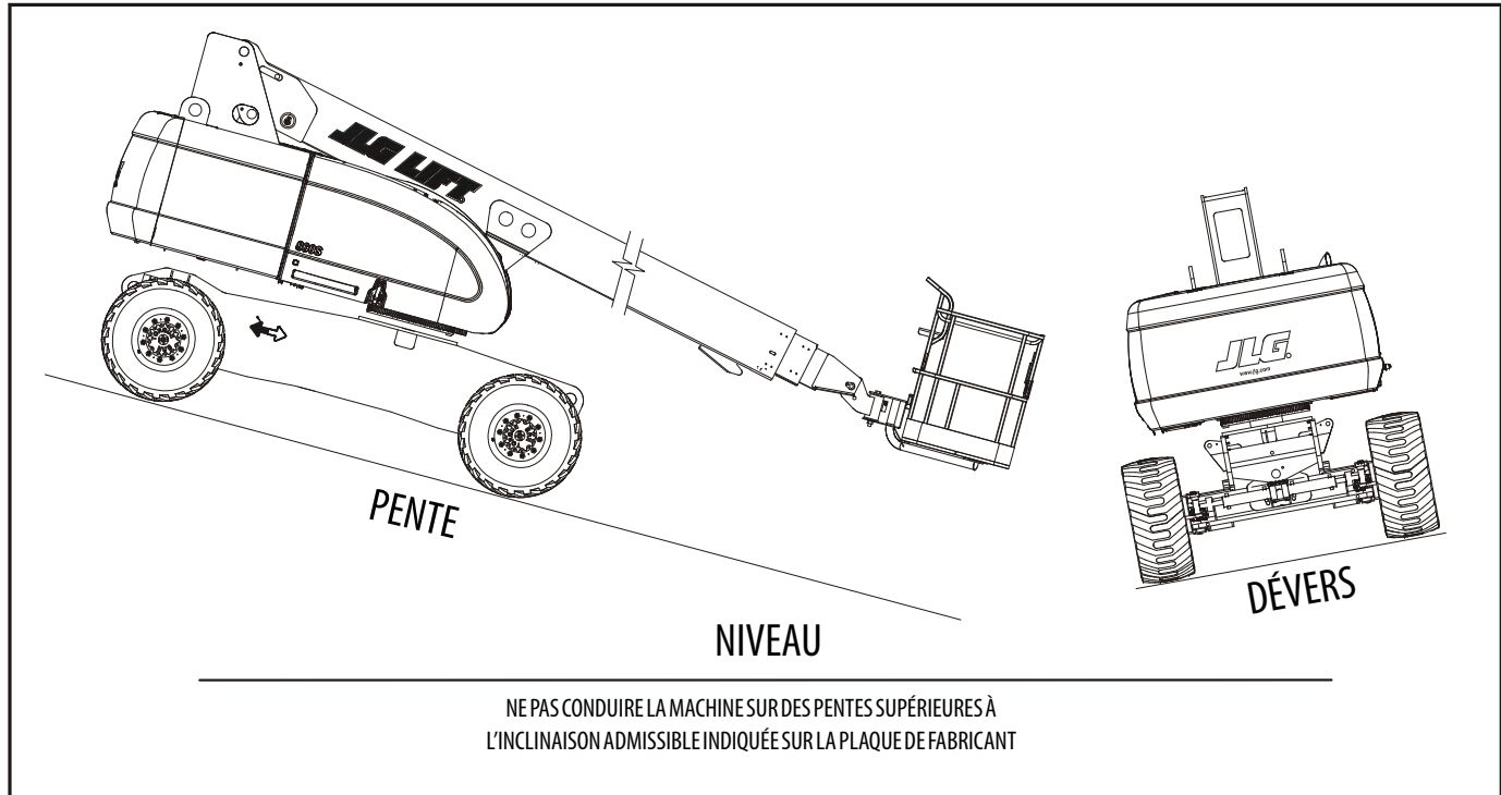
Figure 4-4. Pente et dévers
