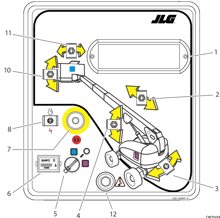
Figure 3-2. Console de commande au sol – 800S avec MSSO
