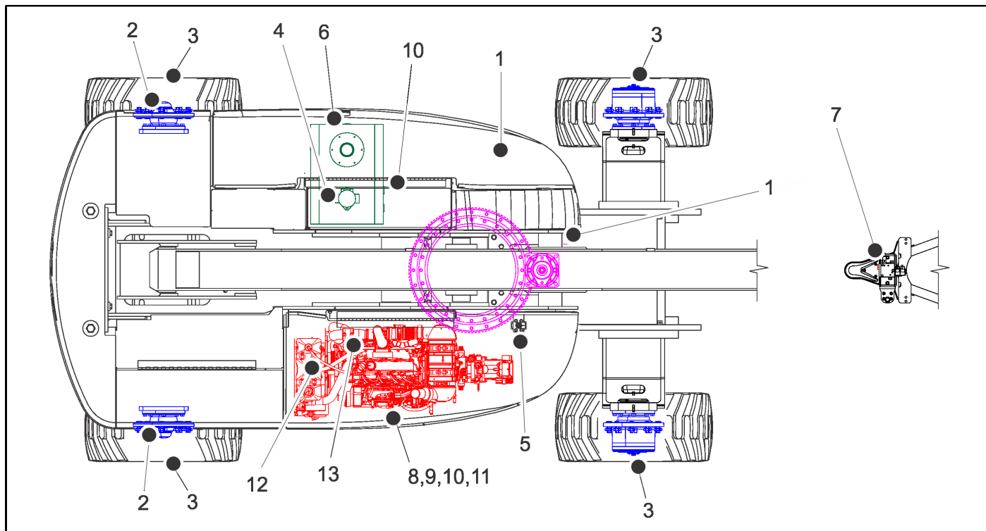
Figure 7-4. Schéma de lubrification et de maintenance
