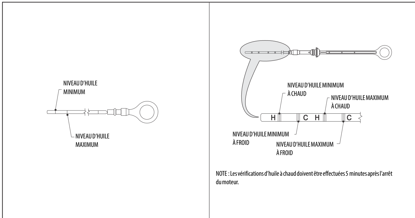
Figure 7-5. Jauge d'huile de moteur Deutz 2011
