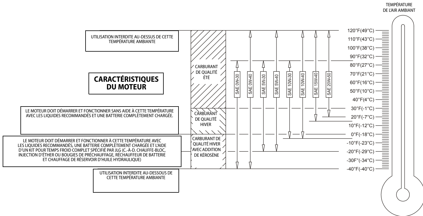
Figure 7-2. Caractéristiques de température de fonctionnement du moteur – Deutz – Fiche 1 de 2
